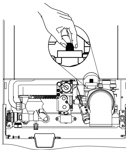
13. attēls. Atgaisošanas ventiļa atvēršana
