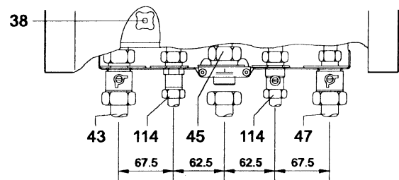
7.att. Montāžas plate
