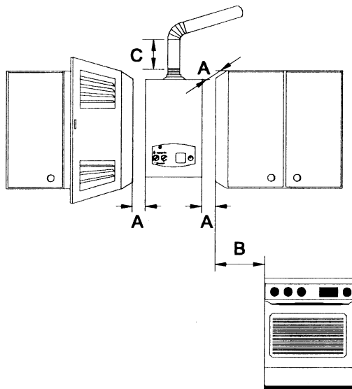
6.att. Minimālie montāžas izmēri
