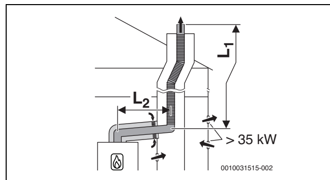
Att. 20 Elastīga dūmgāzu novadišanas sistēma atbilstoši B 33 šahtā ar no telpas gaisa atkarīgu gaisa pievadīšanu caur koncentrisku gaisa pievadīšanu / dūmgāzu novadišanu uzstādīšanas telpā
