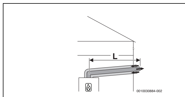
Att. 8 Horizontāli koncentriska gaisa pievadišana / dūmgāzu novadīšana atbilstoši C 13x caur ārsienu
