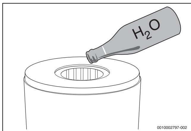
Att. 63 Ar ūdeni izskalot katla bloku
