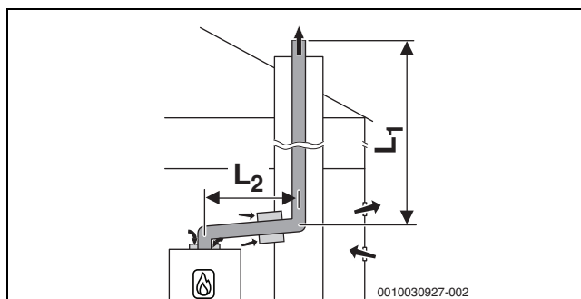
Att. 17 Stingra dūmgāzu novadišanas sistēma atbilstoši B 23p /B 53p ar no telpas gaisa atkarīgu gaisa pievadišanu iekārtai un koncentrisku savienojuma pāreju starp uzstādīšanas telpu un šahtu
