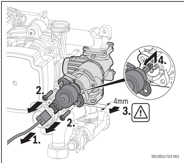
Att. 82 Demontēt trīsvirzienu vārsta motoru (variants ar skrūvēm)
