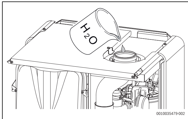
Att. 34 Kondensāta sifona uzpilde ar ūdeni
