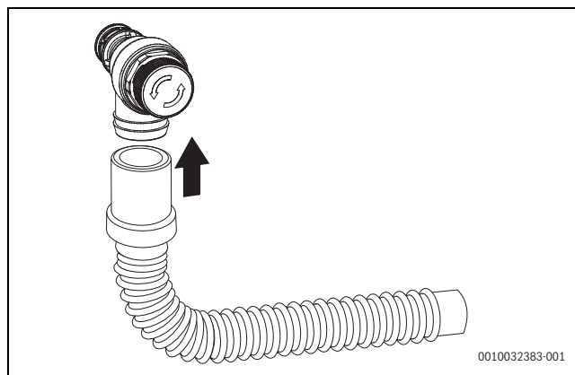
Att. 30 Drošības vārsta (apķure) šļūtenes montāža
