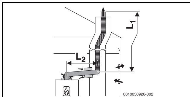
Att. 18 Elastīga dūmgāzu novadišanas sistēma atbilstoši B 23p /B 53p ar no telpas gaisa atkarīgu gaisa pievadišanu iekārtai un koncentrisku savienojuma pāreju starp uzstādīšanas telpu un šahtu
