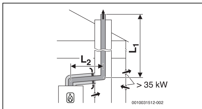
Att. 19 Stingra dūmgāzu novadišanas sistēma atbilstoši B 33 šahtā ar no telpas gaisa atkarīgu gaisa pievadīšanu caur koncentrisku gaisa pievadīšanu / dūmgāzu novadišanu uzstādīšanas telpā
