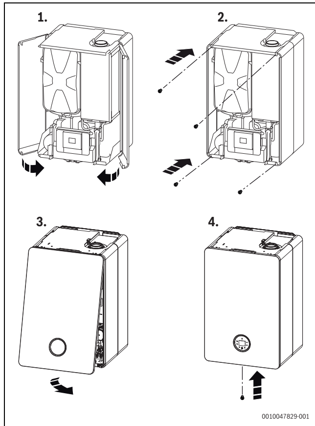
Att. 41 Uzmontēt apšuvumu
