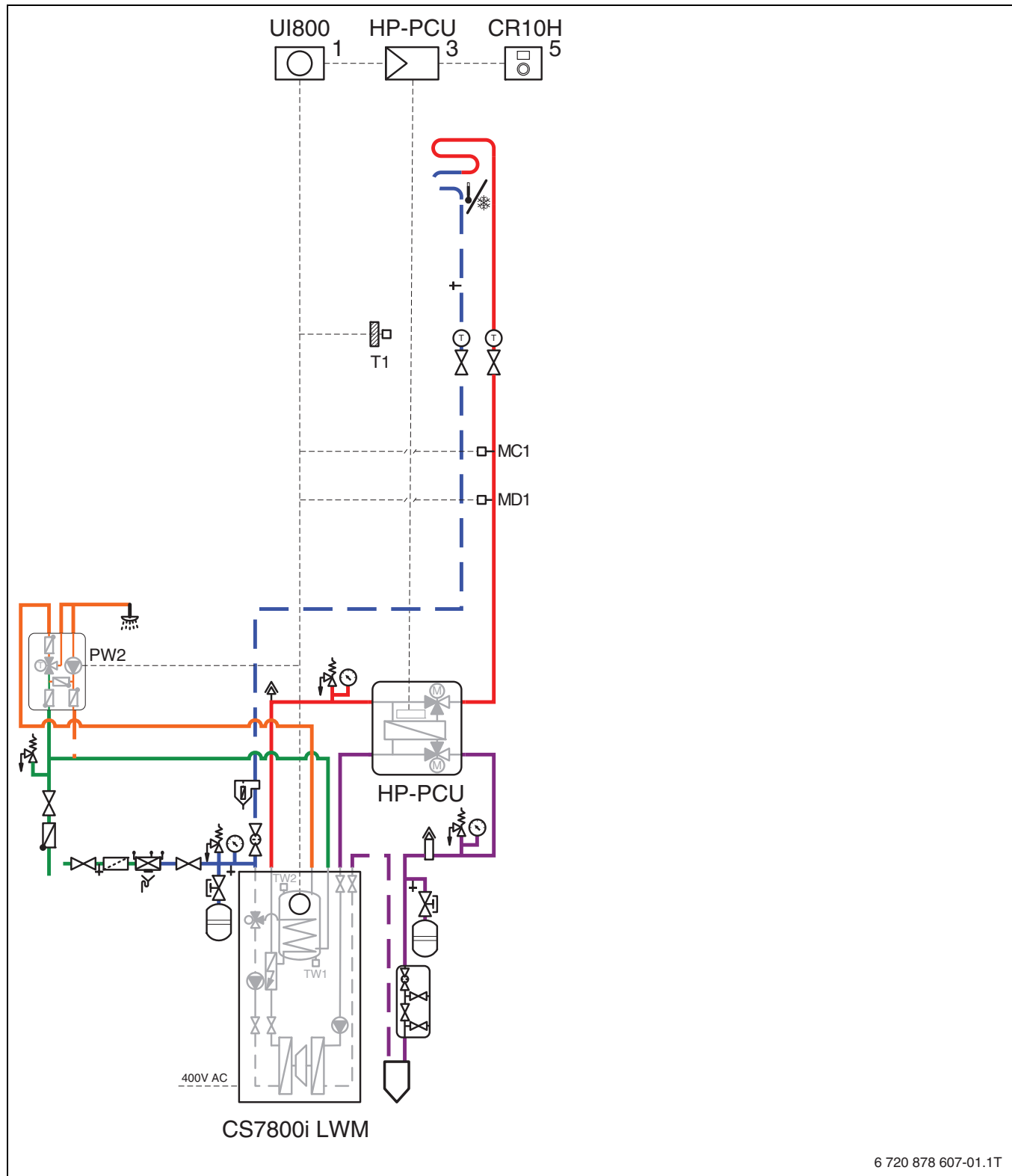
Рис. 11 Стандартный монтаж (без байпаса и бака-накопителя) со станцией пассивного охлаждения
