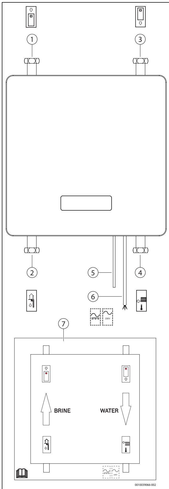
Рис. 4 Подключения к станции пассивного охлаждения
