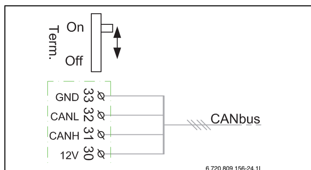
Рис. 10 Терминирование CAN-BUS
