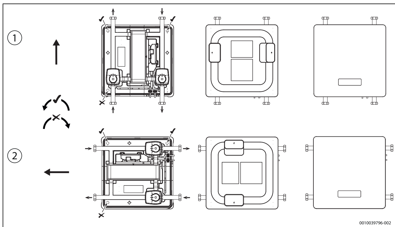
Рис. 5 Вертикальный или горизонтальный монтаж
