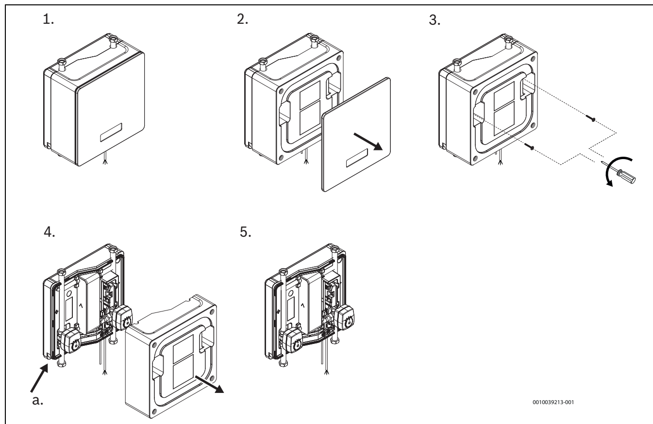
Рис. 6 Подготовка станции охлаждения для настенного монтажа
