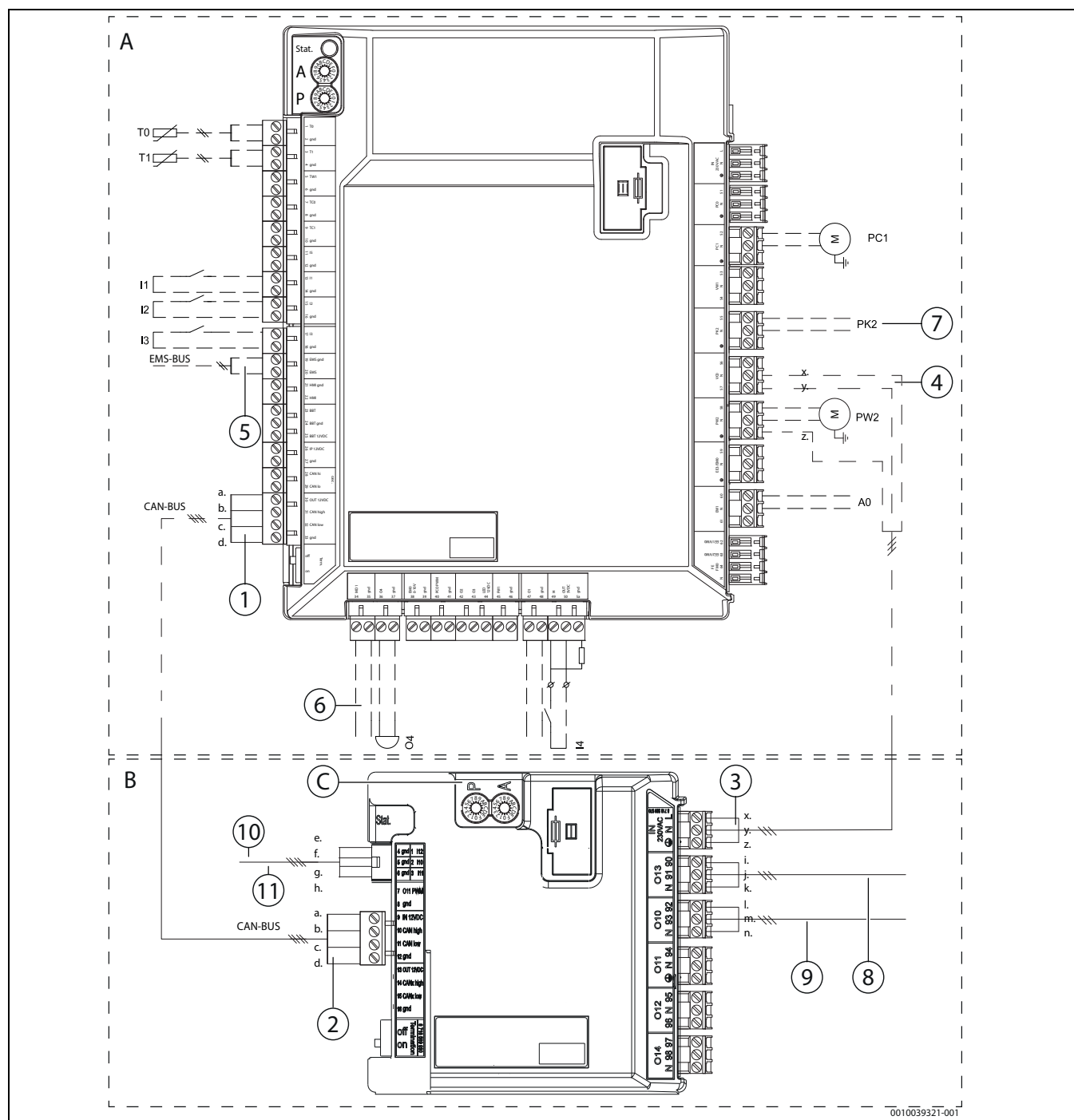
Рис. 9 Схема соединений расширительной электронной платы (станция охлаждения) и монтажной электронной платы (тепловой насос)
